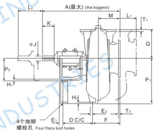
TL(R)系列脱硫泵安装尺寸图 Installation Dimension Diagram of TL(R) FGD Pump
