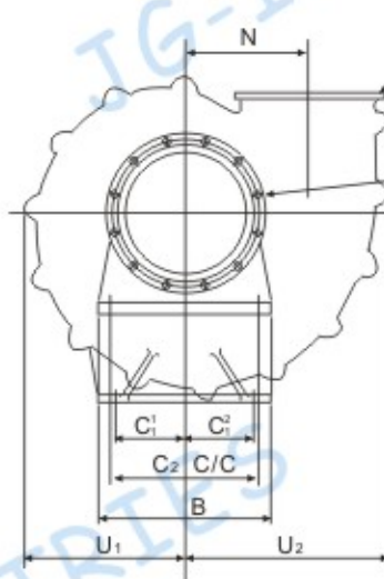
TL(R)系列脱硫泵安装尺寸图 Installation Dimension Diagram of TL(R) FGD Pump
