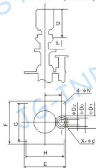
直接传动 Direct Coupled Drive
