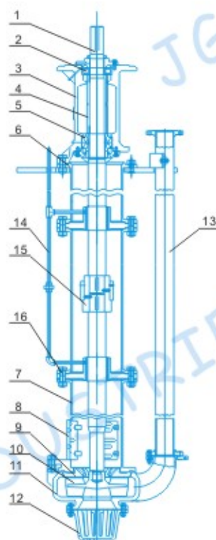
加长型 Extension Type
