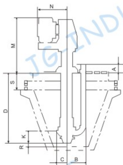
皮带传动 Belt Drive
