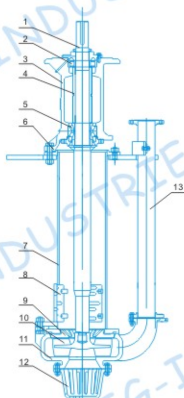
标准型 Standard Type
